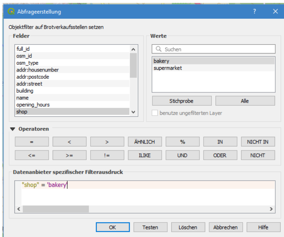
Abbildung 21. Objekte filtern
