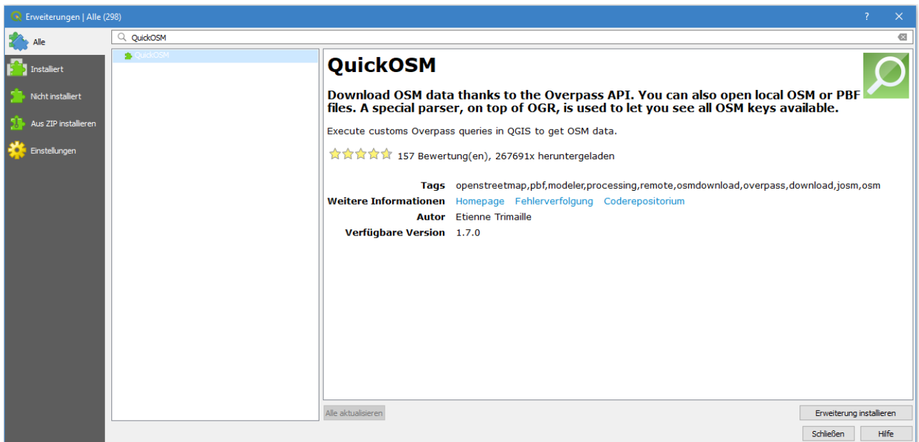
Abbildung 8. QuickOSM Installation
